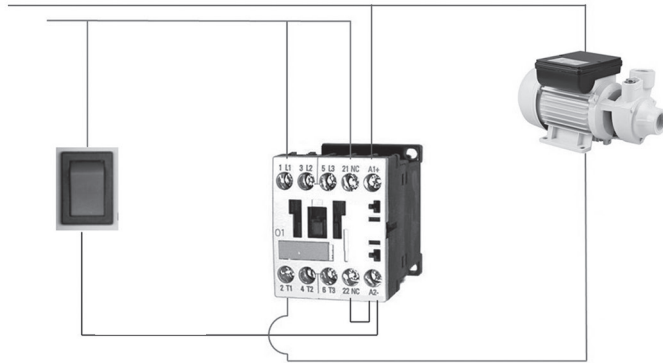
Demonstrativo com bomba monofásica e contator Fase+Neutro com chave liga (para desligar o acionamento deve ser feito diretamente no disjuntor)
